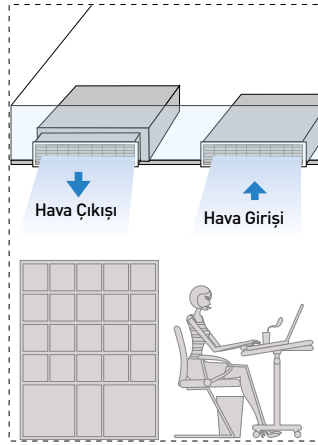
3 Yandan Besleme Altan Geri Dönüş
