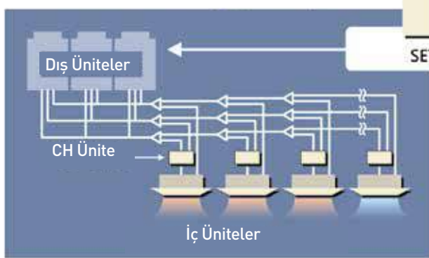
Isı geri kazanım çalışması sistemi kullanıldığı zaman
