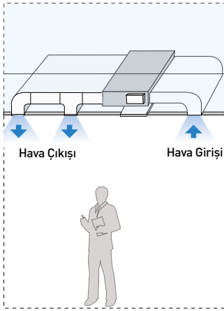
1 Tavandan Besleme
