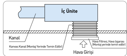
(Hava Taban Giriş Montaj Şeması)
