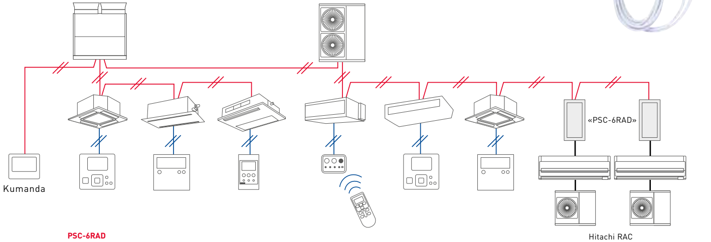
Sistem Yapılandırması Örneği
