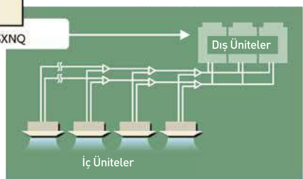
2 borulu geçiş çalışması sistemi kullanıldığı zaman
