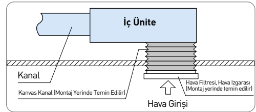
(Hava Tabanı Giriş Montaj Şeması)
