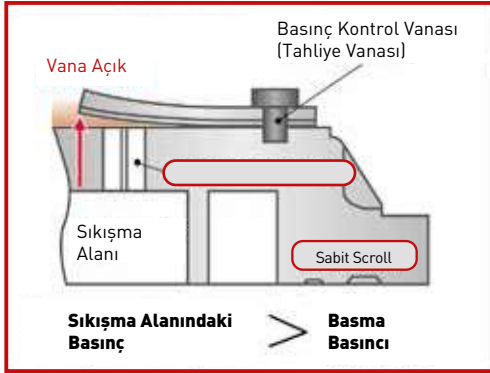
Basma Basıncı Alanı
