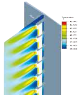
Hava Dağıtımı
