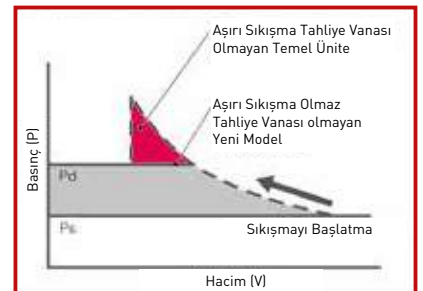
Teorik PD diyagramı
