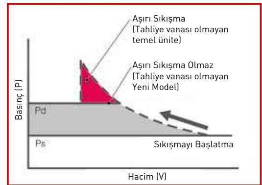
Teorik PD diyagramı
